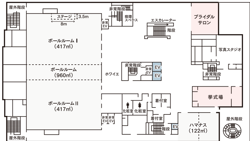
3階 3rd floor [天井高 ボールルーム6.0m ハマナス2.7m]
